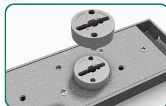
Guidachiave componibile di 8 mm
